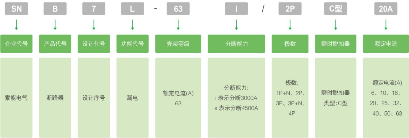
SNB7L 小型漏电断路器
